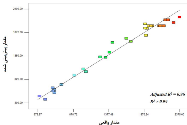
شکل 1. مقدار پیش‌بینی شده - مقدار واقعی
