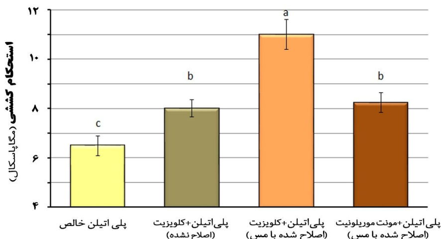
شکل 5. تأثیر افزودن انواع نانوذرات خاک رس اصلاح شده با فلز مس بر استحکام کششی فیلم پلی اتیلنی
