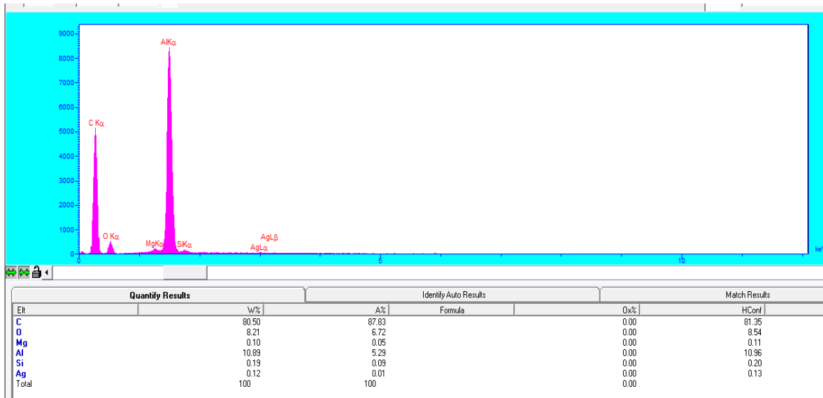
شکل 4. عناصر تشکیل دهنده مجموع قوطی و پوشش داخلی
