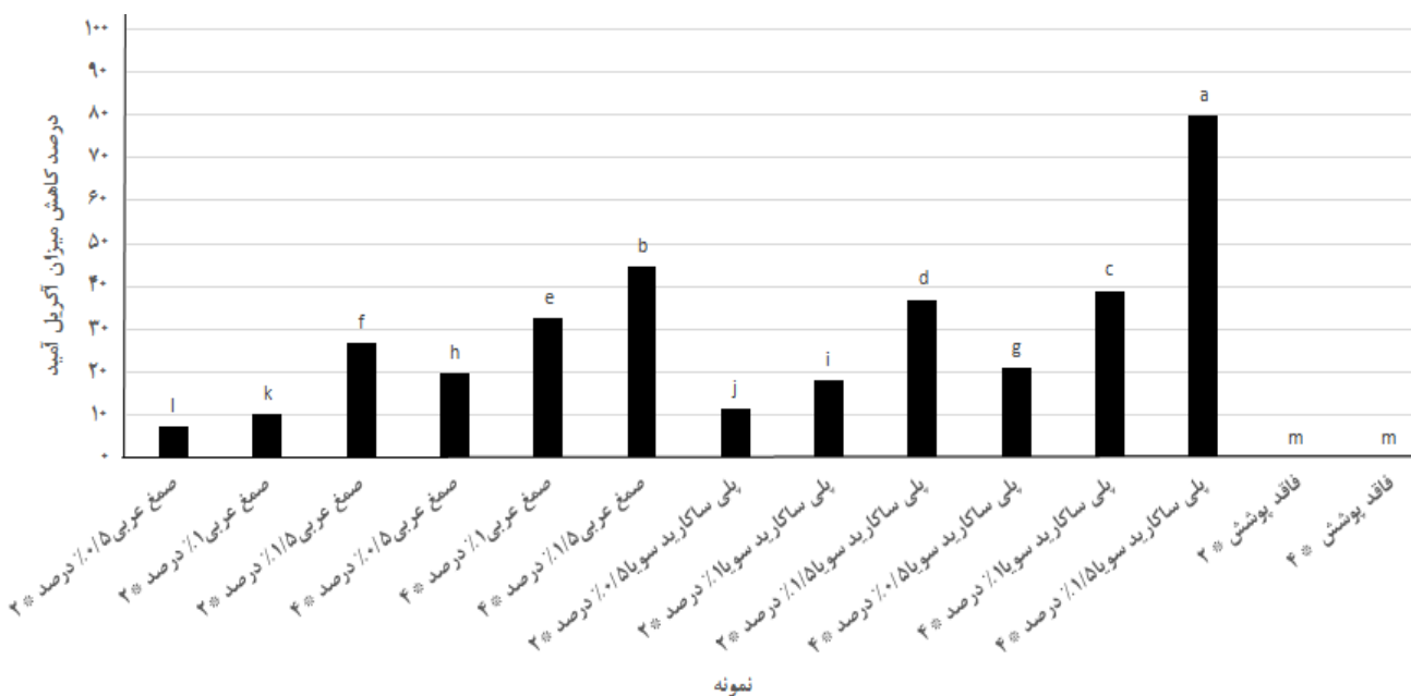
نمودار 1. اثر پوشش‌دهی بر میزان کاهش تشکیل آکریل‌آمید در نمونه‌های چیپس سیب‌زمینی سرخ‌شده (درصد)
