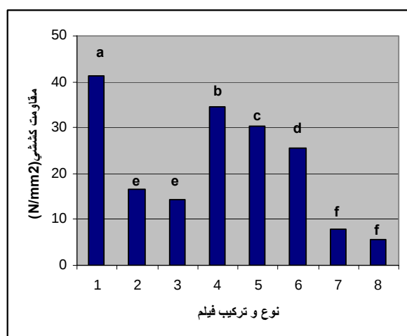
شکل ۱- مقایسه مقاومت کششی فیلم‌های متیل سلولز
