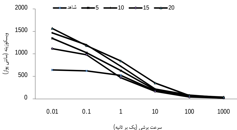
شکل 4. تغییرات ویسکوزیته ظاهری به سرعت برشی در نمونه‌های دوج حاوی غلظت‌های مختلف آلوه ورا
