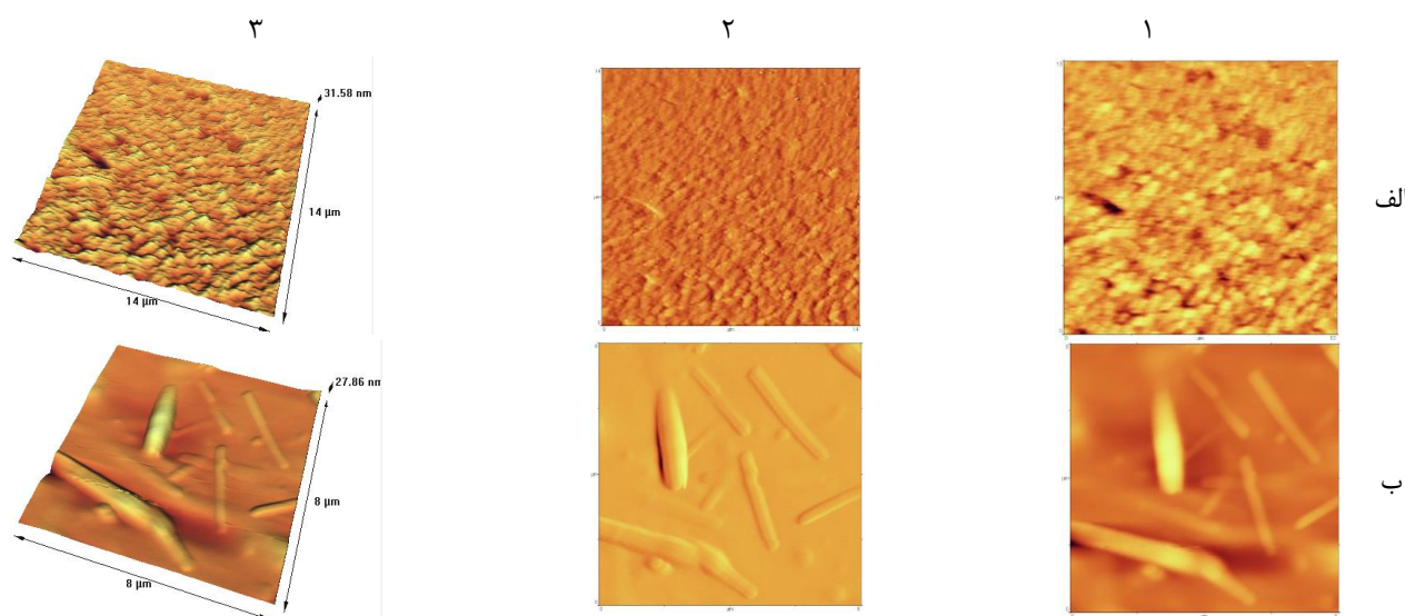
شکل ۵. الف- تصاویر AFM از نانوذرات آلبومین حاوی کورکومین در سو سپانسیون، در pH ۷؛ و ب- تصاویر AFM از سو سپانسیون نانوذرات آلبومین حاوی کورکومین پایدارشده با گلو تار آلدئید، پس از ده روز نگهداری، توپوگرافی (۱) سطحی دو بعدی؛ (۲) نوسانی و (۳) سه بعدی
