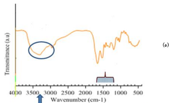
شکل ۴. طیف IR (الف) کورکومین؛ (ب) آلبومین؛ (ج) نانوذرات آلبومین شاهد؛ (د) نانوذرات آلبومین پیوندشده با گلو تار آلدئید و (ه) طیف IR نانوذرات آلبومین پیوند شده با اسید تانیک (دایره آبی و گروه به ترتیب اعداد موج بر حسب \text{cm}^{-1} ) در ناحیه هیدروکسیل ۳۳۲۰ و آمیدی (۱۶۶۴-۱۵۳۴-۱۲۴۲) را نشان می‌دهند.
