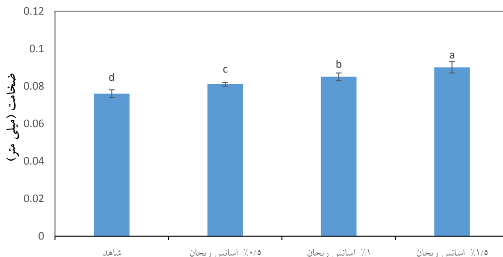
نمودار ۱. اثر افزودن غلظت‌های مختلف اسانس ریحان بر ضخامت فیلم بر پایه صمغ دانه اسفرزه (حروف انگلیسی متفاوت نشان‌دهنده اختلاف معنی‌دار آماری در سطح اطمینان ۹۵٪ می‌باشد).
