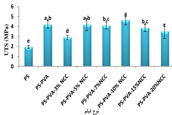
شکل ۴. اثر PVA و NCC بر روی UTS فیلم‌های نشاسته نرم شده (PS)، نشاسته نرم شده- پلی وینیل الکل (PS-PVA) و نانوکامپوزیت‌های PS-PVA حاوی مقادیر مختلفی از NCC (اعداد مشابه در سطح ۰.۵٪ تفاوت معنی‌داری با هم نشان می‌دهند)
