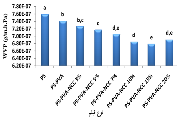
شکل ۶. نمودار عبور بخار آب از فیلم نشاسته نرم شده (PS)، نشاسته نرم شده و پلی وینیل الکل (PS-PVA)، نانوکامپوزیت‌های نشاسته نرم شده و پلی وینیل الکل حاوی مقادیر مختلفی از NCC (اعداد مشابه در سطح ۰.۵٪ تفاوت معنی‌داری با هم نشان می‌دهند)
