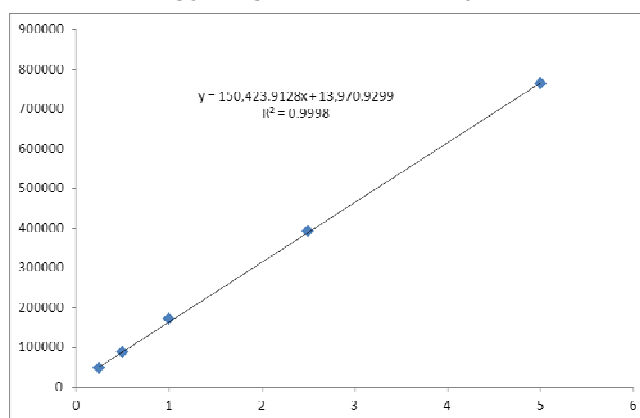
شکل ۳. نمودار خطی کالیبراسیون بنزو (a,h) پیرن، مقدار بر حسب ppb
