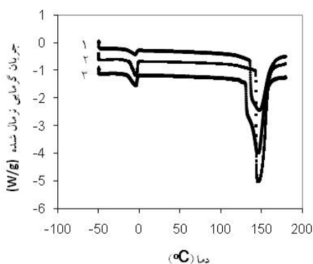
شکل 4. دمانگاشت‌های گرماسنج پویشی تفاضلی برای نان تست بسته‌بندی شده در فیلم‌های نانویی و فیلم معمولی پس از 4 روز نگهداری در 25 درجه سانتی‌گراد
