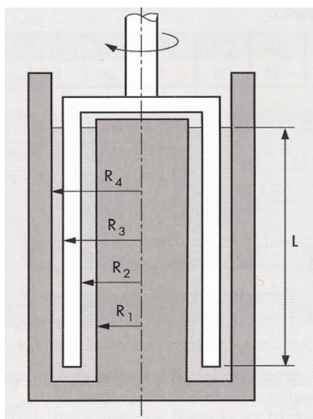
شکل ۱- رئومتری استوانه هم محور دوگانه
