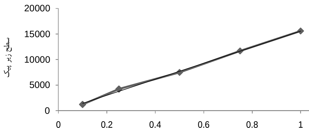
شکل 2. منحنی کالبراسیون تایلوزین
