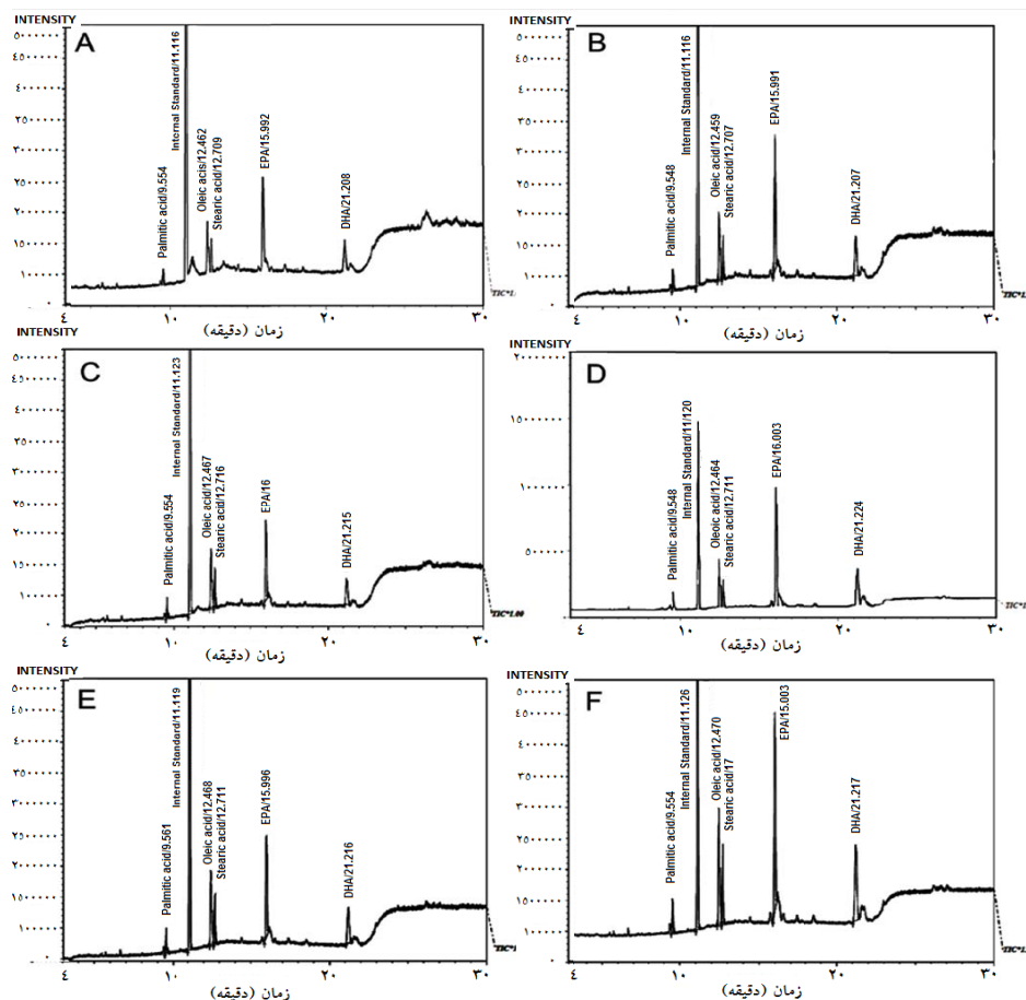
شکل ۳. آنالیز کروماتوگرافی گازی A: نمونه استاندارد، کمپلکس‌های کازئینات-پکتین با نسبت‌های B: (۰/۲-۱)، C: (۰/۲-۰/۵)، D: (۰/۴۵-۱)، E: (۰/۴۵-۰/۵) و F: (۰/۷-۱)
