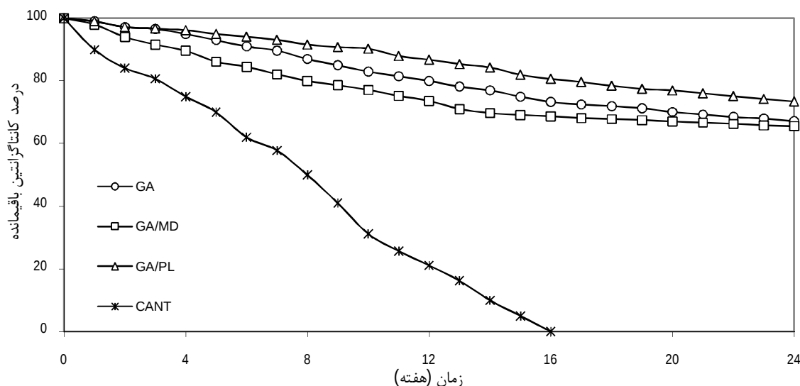
شکل 2. مقایسه میزان پایداری کانتاگزانتین موجود در ریزکپسول‌ها طی 24 هفته نگهداری در دمای 25°C GA صمغ عربی، MD مالتودکستری، PL پولولان، CANT کانتاگزانتین بدون پوشش
