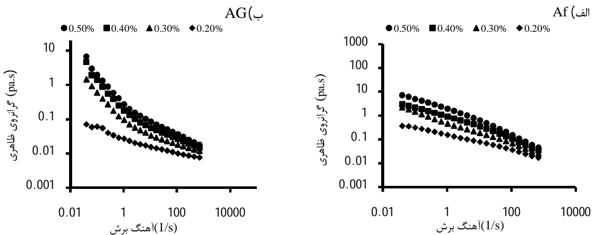
نمودار 2. اثر غلظت (0/2 تا 0/5 % با مقیاس وزنی/وزنی) و نوع صمغ کتیرا (الف و ب) بر وابستگی گرانروی ظاهری به آهنگ برش در نمونه های امولسیون در دمای 25°C
