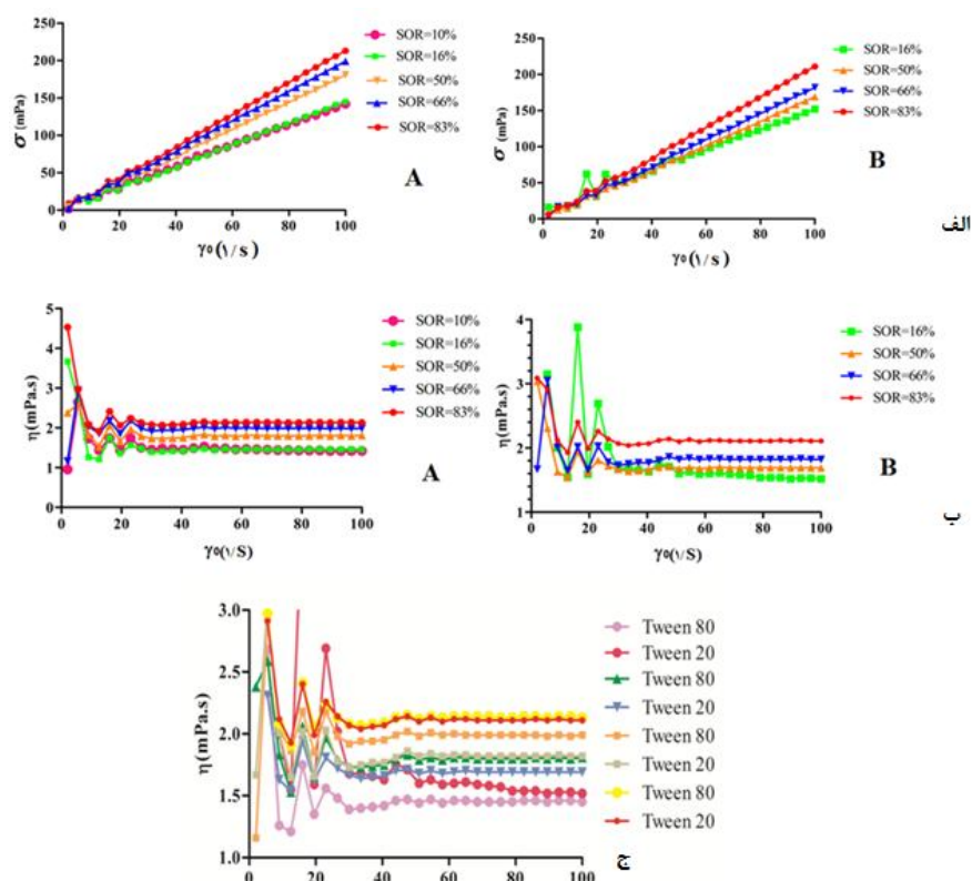
شکل 5. الف- نمودار تنش برشی - سرعت برشی برای نمونه های حاوی غلظت های مختلف سورفاکتانت (توپین 80: A - توپین 80 - نمودار ویسکوزیته و سرعت برشی نمونه های تهیه شده در غلظت های مختلف سورفاکتانت توپین 80 (A) و توپین 20 (B) در مقدار ثابت 10 گرم آب، ج- نمودار ویسکوزیته و سرعت برشی نمونه های توپین 80 و 20 در غلظت های مختلف سورفاکتانت های 16% (دایره)، 50% (مثلث)، 66% (مربع)، 83% (شش ضلعی)
