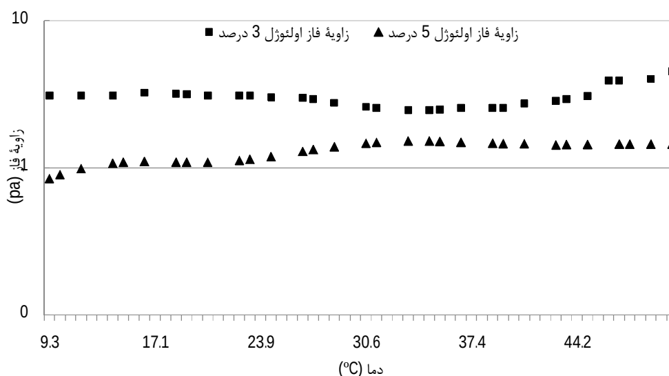
شکل 5. زاویه فاز (مدول تانژانت) اولئوژل‌های روغن آفتابگردان
