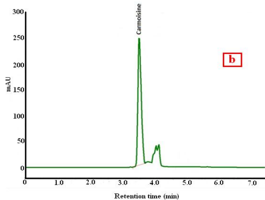
شکل 4. کروماتوگرام نمونه ژله A قبل (a) و بعد از اسپایک (b) 250 \mu\text{g L}^{-1} از محلول استاندارد کارموزین
