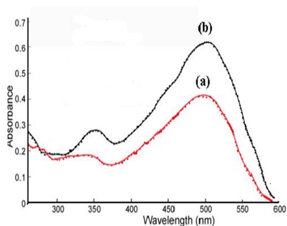
شکل 3. طیف مرئی نمونه ژله A قبل (a) و بعد از اسپایک (b) 250 \mu\text{g L}^{-1} از محلول استاندارد کارموزین
