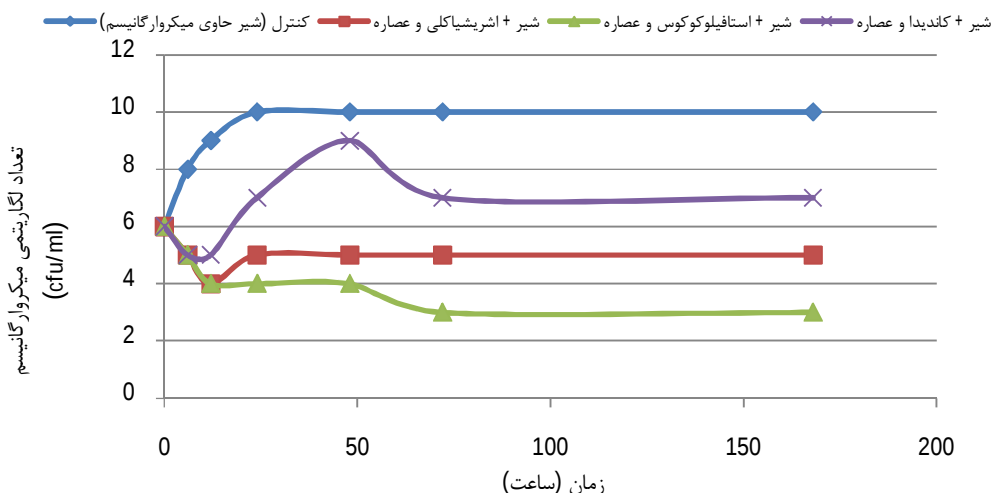
نمودار 1. تعداد لگاریتمی اشیریشیاکلی، استاف و کاندیدا بر حسب زمان در دمای 37°C برای باکتری‌ها و 25°C برای قارچ
