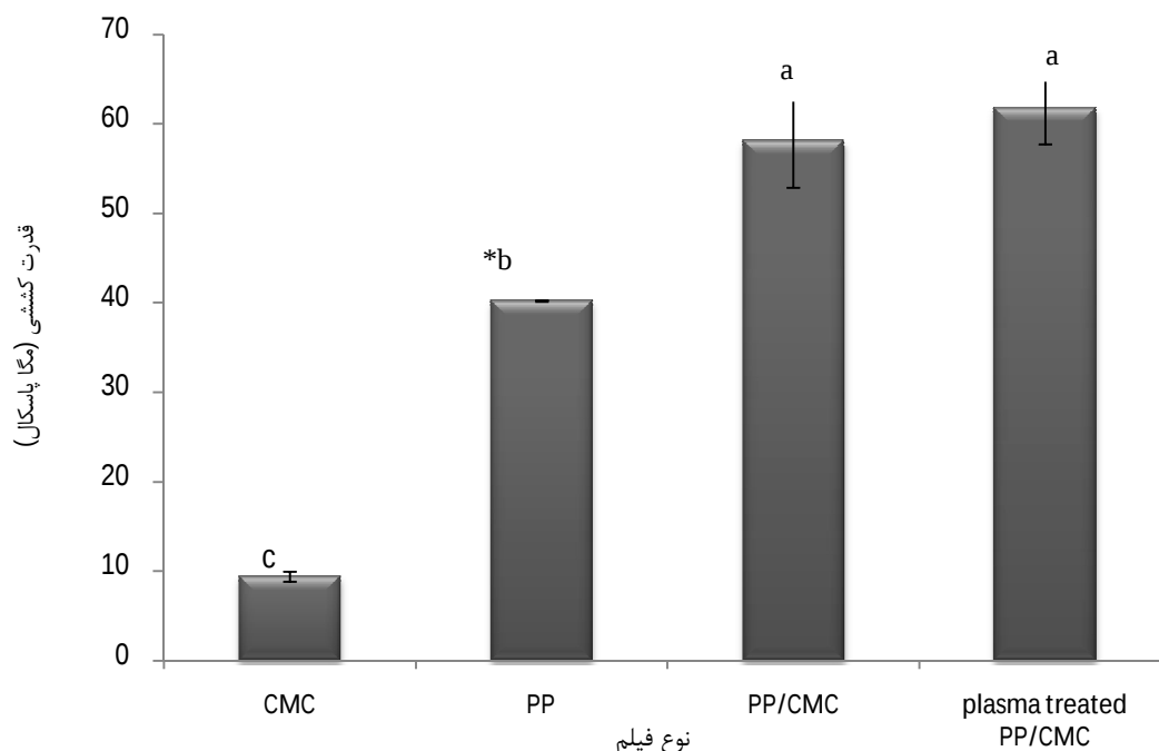
شکل 1. قدرت کششی (مگا پاسکال) در فیلم خوراکی کربوکسی متیل سلولز (CMC)، فیلم پلی پروپیلن (PP)، فیلم دولایه ی PP/CMC غیر تیمار شده و تیمار شده با پلاسما
