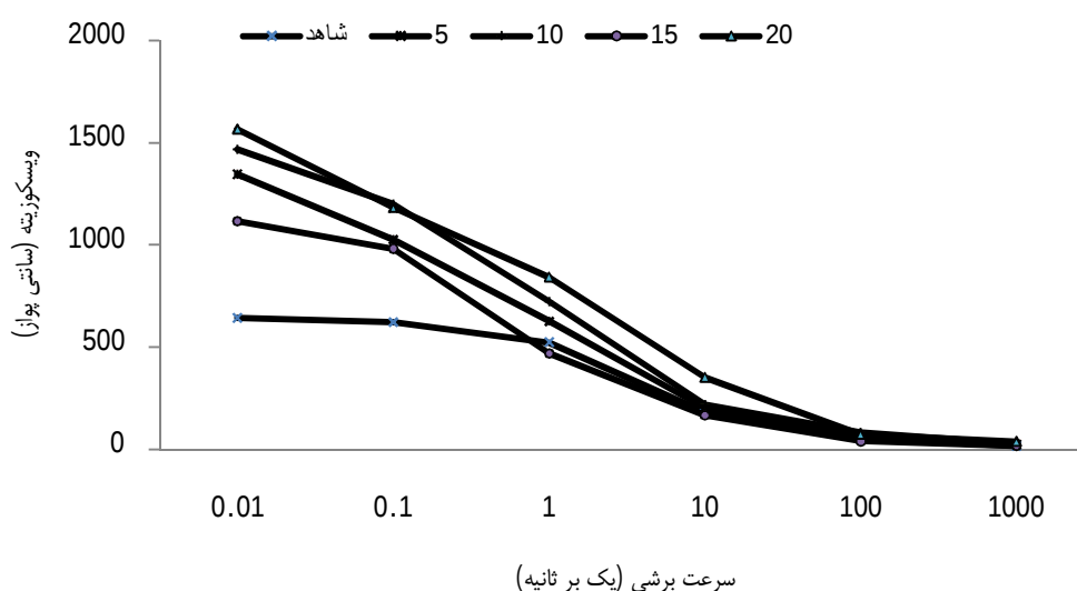
شکل 4. تغییرات ویسکوزیته ظاهری به سرعت برشی در نمونه‌های دوج حاوی غلظت‌های مختلف آلئوئه ورا
