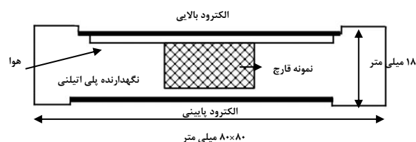
شکل ۱. تصویر نگهدارنده نمونه از نمای رو به رو
