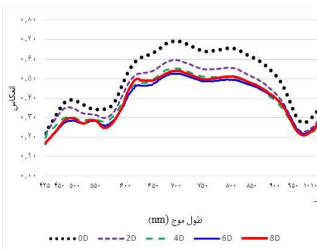
شکل ۱. نمودار طیفی فیله‌های ماهی گوزیوم دم رشته‌ای طی ۸ روز
