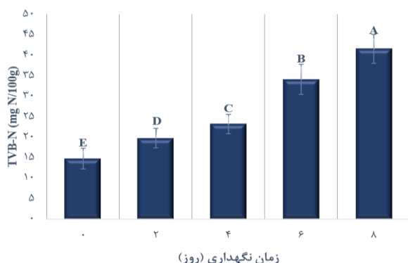
شکل ۲. شاخص بازهای نیتروژنی فرار در نمونه‌های ماهی گوزیوم دم رشته‌ای
