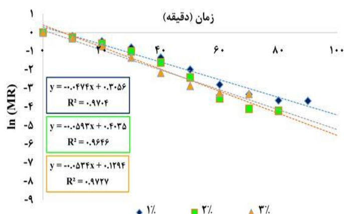
شکل ۳. تأثیر غلظت اولبومین بر ضریب انتشار مؤثر رطوبت در دمای ۷۰ درجه سلسیوس و ضخامت ۳ میلی‌متر
