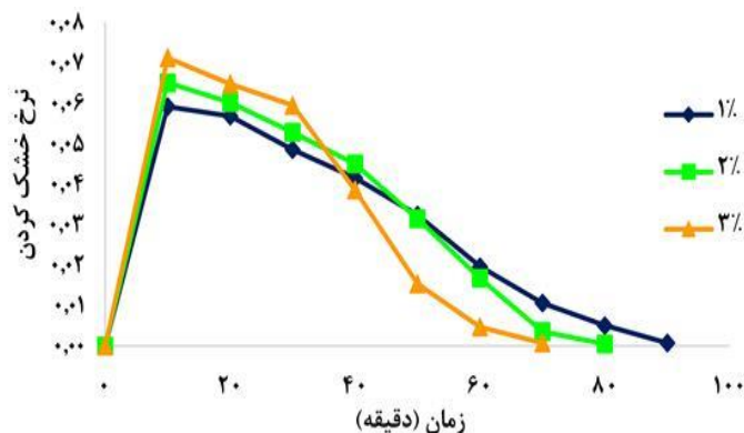
شکل ۲. تأثیر غلظت اولبومین بر نرخ خشک کردن در دمای ۷۰ درجه سلسیوس و ضخامت ۳ میلی‌متر
