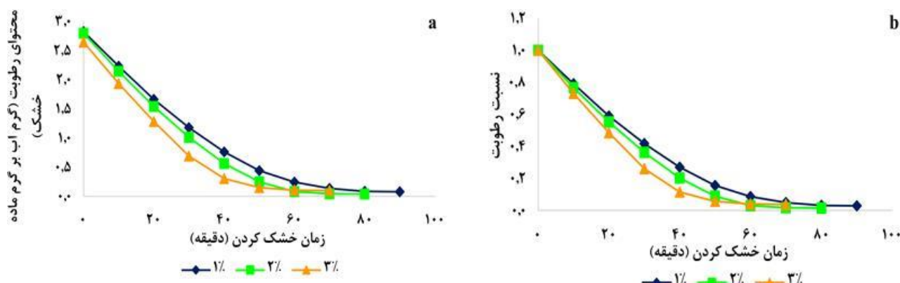
شکل ۱. تأثیر غلظت اولبومین بر منحنی‌های خشک کردن کف پوره موز نارس (محتوای رطوبت و نسبت رطوبت) در دمای ۷۰ درجه سلسیوس و ضخامت ۳ میلی‌متر
