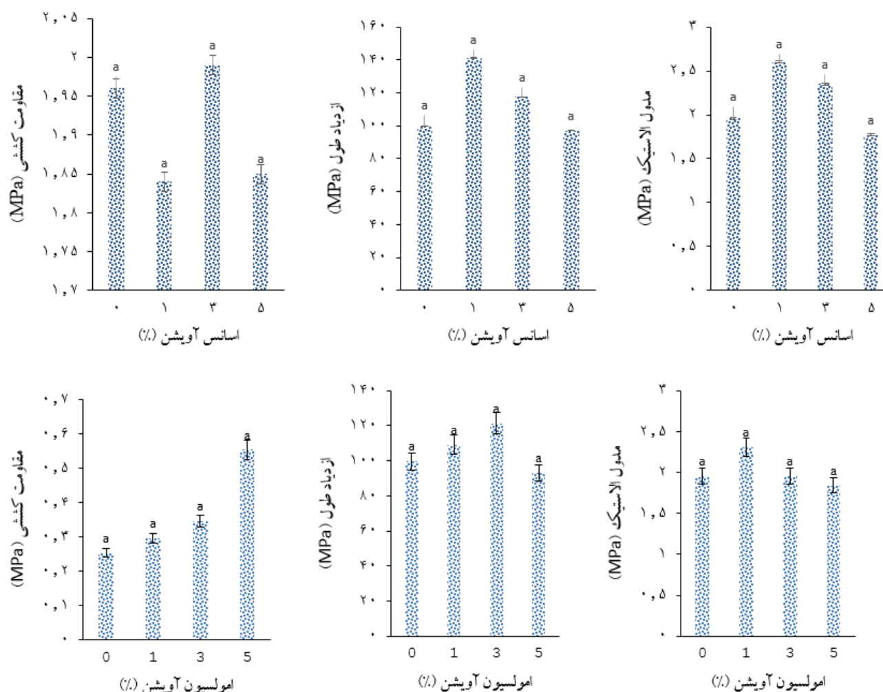
شکل ۵. منحنی مقایسه میانگین اثر (a) اسانس و (b) امولسیون آویشن بر روی (۱) مقاومت کششی (۲) ازدیاد طول تا حد پاره شدن (۳) مدول الاستیک فیلم‌های تولیدی
