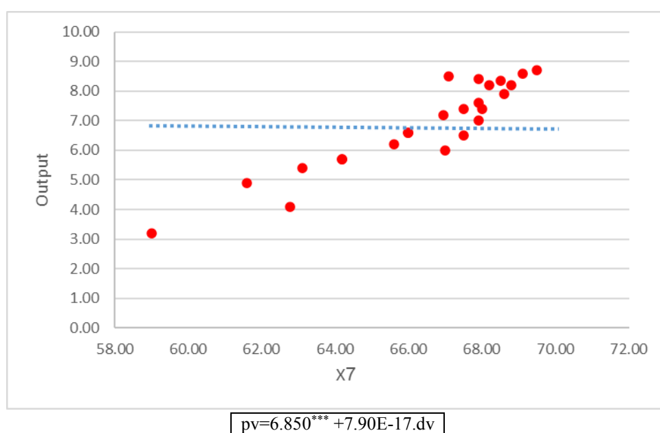
شکل ۸. تحلیل حساسیت پارامتر درصد سختی (X7) در مدل پیش‌بینی GPR
