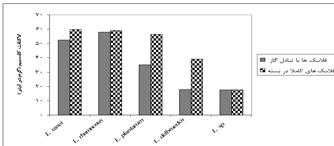
شکل ۲- تولید لاکتات کلسیم توسط لاکتوباسیل‌های مختلف در محیط دارای ۱۰۰g/l گلوکز در شرایط متفاوت هوادهی
