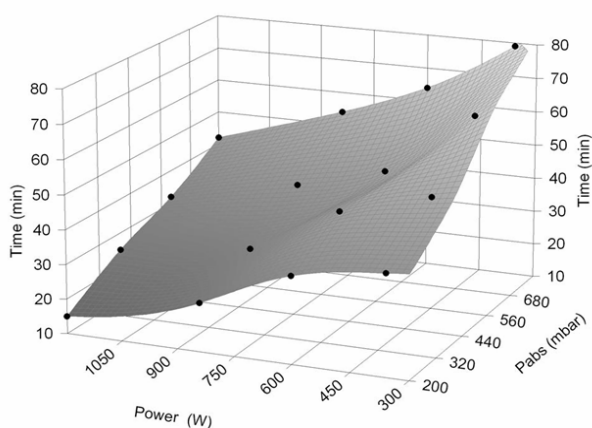
شکل ۳- تأثیر هم‌زمان توان مایکروویو و فشار مطلق خشک کن مایکروویو-خلأ بر مدت زمان خشک شدن میوه آلبالو
