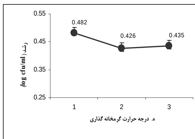
شکل ۲- تأثیر سطوح مختلف متغیرهای فیزیکی و شیمیایی محیط کشت بر شمارش میکروبی باکتری لاکتوباسیلوس / اسیدوفیلوس طی مدت گرمخانه گذاری. سطوح ۱ تا سه هر متغیر مطابق مقادیر تعریف شده در جدول ۱ است. (الف) شیر خشک بدون چربی؛ (ب) پودر آب پنیر؛ (ج) درصد تلقیح لاکتوباسیلوس / اسیدوفیلوس؛ (د) میزان تلقیح کشت آغازگر ماست؛ (ه) دمای گرمخانه گذاری
