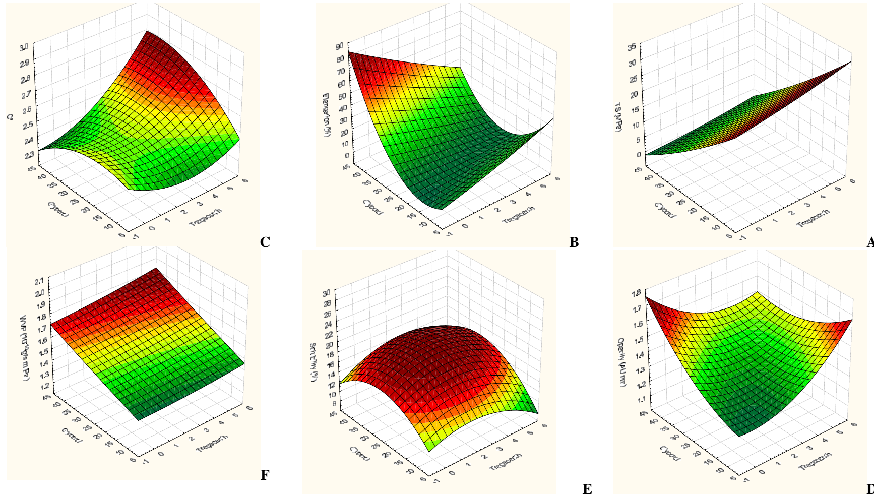
شکل ۱- چند نمونه از گراف‌های RSM. در این گراف‌ها اثر متقابل ثعلب و گلیسرول روی ویژگی‌های مختلف فیلم خوراکی نشان داده شده است.
