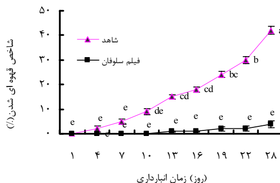
شکل ۲. تغییرات شاخص قهوه‌ای شدن از گیل ژاپنی پس از ۲۸ روز انبارداری در دمای ۷°C
