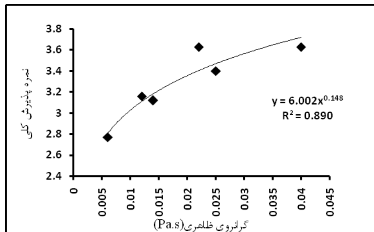
نمودار ۴. رابطه ارزیابی حسی با گرانیوی ظاهری (در سرعت برش 50 \text{ s}^{-1} ) نمونه‌های شیر خرما
