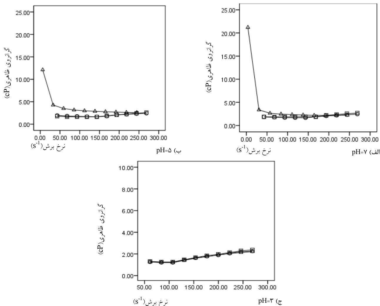
شکل ۲. گرانیوی ظاهری محلول‌های صمغ ژلان در مقابل نرخ برش
