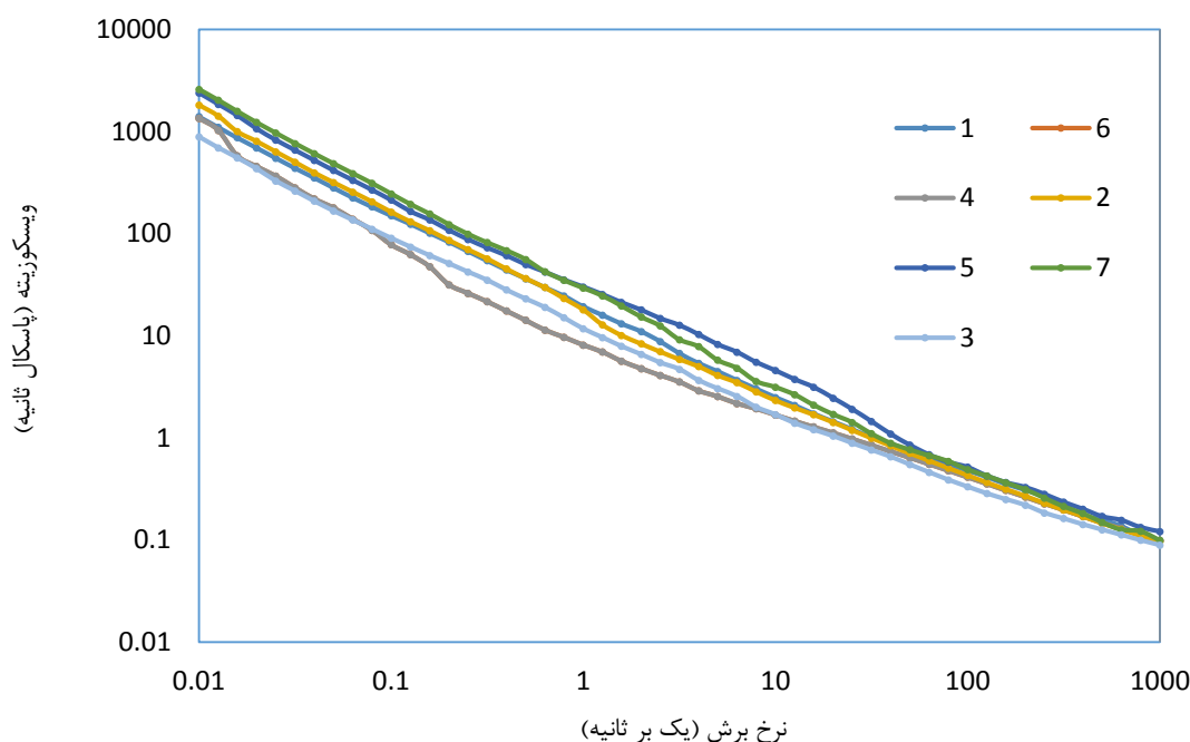
شکل ۳. تغییرات ویسکوزیته نسبت به سرعت برش در نشاسته‌ی ذرت تیمار شده با امواج الکترومغناطیس
