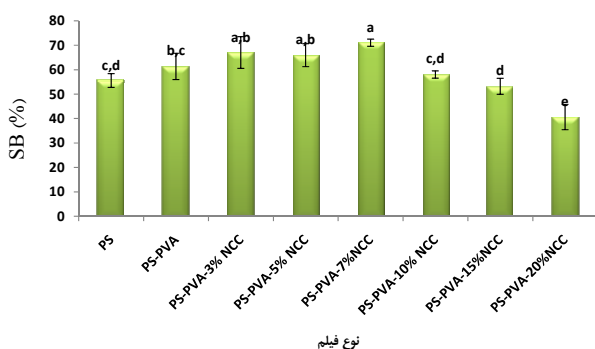
شکل ۵. اثر PVA و NCC بر روی SB فیلم‌های نشاسته نرم شده (PS)، نشاسته نرم شده/ پلی وینیل الکل (PS-PVA) و نانوکامپوزیت‌های حاوی NCC (اعداد مشابه در سطح ۵٪ تفاوت معنی‌داری با هم نشان می‌دهند)
