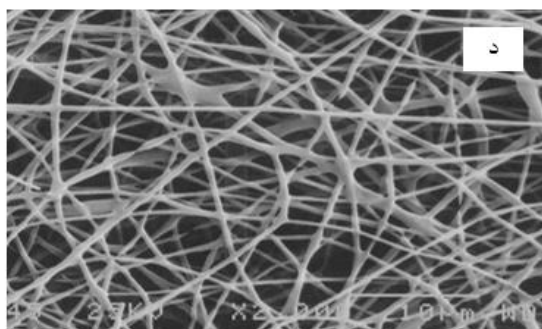
شکل ۵. تصاویر میکروسکوپ الکترونی روبشی از سطح فویل آلومینیوم پوشش‌دهی شده با محلول صمغ آنغوزه در حلال استیک اسید در غلظت ۲۰ درصد با شرایط دستگاهی بهینه
