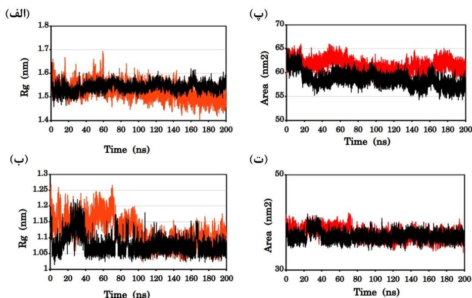
شکل ۳. نمودار Rg (الف) برای ssRNA (سیاه) و ssRNA-سافرانال (قرمز؛ ب) برای ssDNA (سیاه) و ssDNA-سافرانال (قرمز؛ ت) SASA (پ) برای ssRNA (سیاه) و ssRNA-سافرانال (قرمز)، و (ت) برای ssDNA (سیاه) و ssDNA-سافرانال (قرمز).
