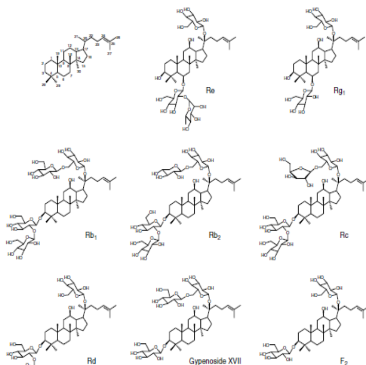
شکل ۲. ساختار چند جینسنوزید معمول در پاناکس (۲۰)
