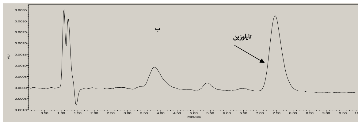
شکل 1. کروماتوگرام الف) استاندارد تایلوزین ( 1 \mu\text{g ml}^{-1} ) ب) تایلوزین اضافه و بازیابی شده از گوشت ( 400 \mu\text{g g}^{-1} )
