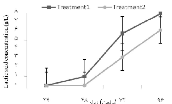
شکل 5. روند تغییرات غلظت اسید لاکتیک طی دوره تخمیر در دو تیمار مختلف در سامانه ناپیوسته خوراک‌دهی شده در دمای 30 درجه سانتی‌گراد و طی مدت 96 ساعت؛ مربع توپر مربوط به تیمار 1 (تخمیر با کنترل pH محیط با سود 1 نرمال) و دایره توپر مربوط به تیمار 2 (تخمیر بدون کنترل pH محیط) است.
