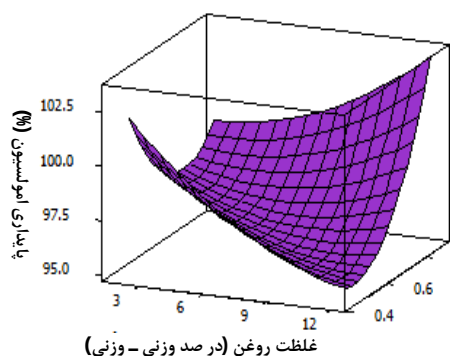
شکل 3. اثر همزمان متغیرهای K_0 و غلظت روغن بر پایداری امولسیون
