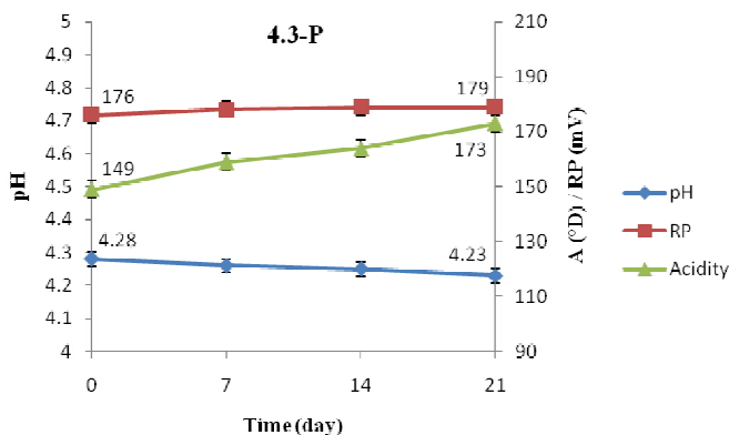
شکل 1. تغییرات pH، اسیدیته قابل تیتر و پتانسیل احیا طی 21 روز نگهداری یخچالی (5°C) در تیمارهای با pH اولیه طبیعی (4/3) و تلقیح شده با سوش‌های پروبیوتیک (A=ل.اسیدوفیلوس، C=ل.کازنی، F=ل.فرمنتوم، FR=روتیری و P=ل.پلنناروم)
