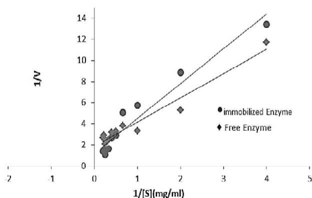
شکل 3. نمودار Lineweaver -Burk مربوط سرعت واکنش آنزیمی در غلظت‌های مختلف سوبسترا
