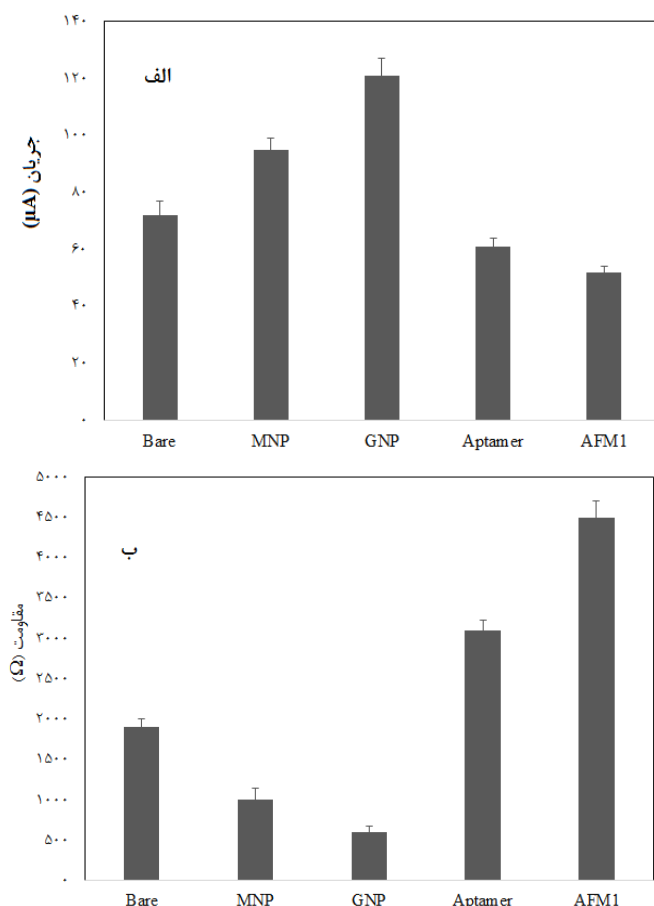
شکل ۱. پیک جریان (الف) و مقاومت انتقال بار (ب) در مراحل مختلف اصلاح الکتروود کاری
