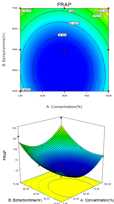
شکل ۶. نمودار دوبعدی (کنتور) و سه‌بعدی تغییرات میزان قدرت احیاء‌کنندگی عصاره‌های اتانولی گیاه بن‌سرخ تحت تأثیر غلظت حلال اتانولی و زمان استخراج (دمای استخراج ۴۰ درجه سانتی‌گراد)
