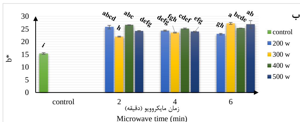
شکل ۵. اثر توان‌ها و زمان‌های متفاوت میکروویو بر b^* در دمای الف. ۱۶۰، ب. ۱۸۰ درجه سانتی‌گراد *حروف غیرمشابه نشان‌دهنده تفاوت معنی‌دار میان نمونه‌ها می‌باشد.
