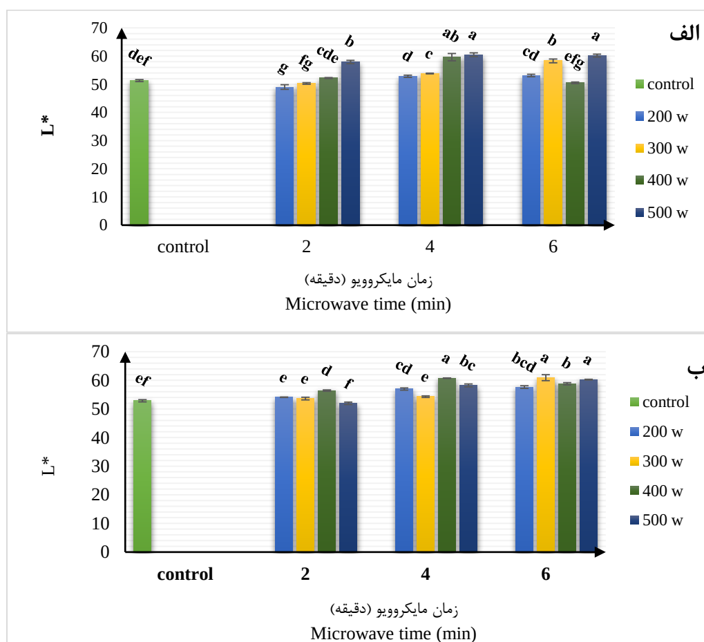
شکل ۳. اثر توان‌ها و زمان‌های متفاوت مایکروویو بر L^* در دمای الف. ۱۶۰، ب. ۱۸۰ درجه سانتی‌گراد
