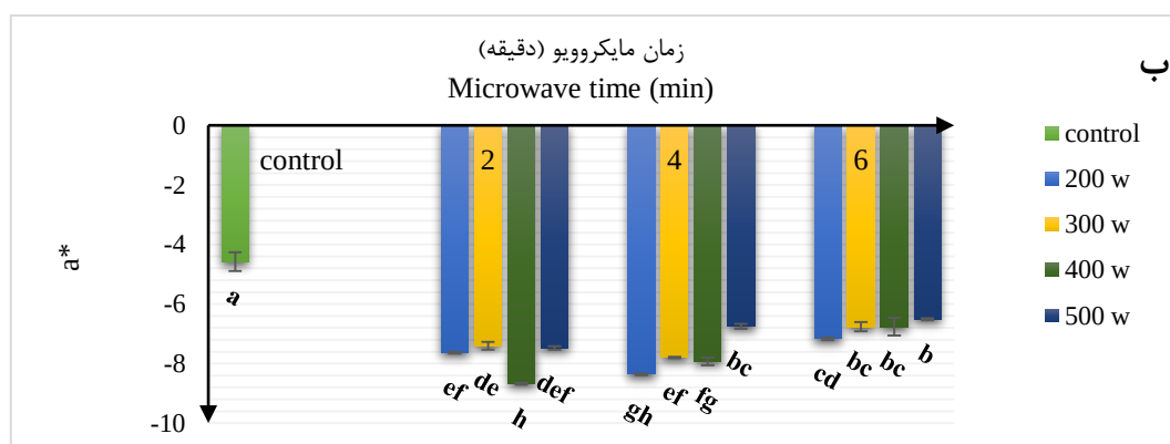
شکل ۴. اثر توان‌ها و زمان‌های متفاوت میکروویو بر a^* در دمای الف. ۱۶۰، ب. ۱۸۰ درجه سانتی‌گراد *حروف غیرمشابه نشان‌دهنده تفاوت معنی‌دار میان نمونه‌ها می‌باشد.
