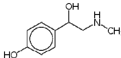
شکل ۳. ساختار سینفرین
