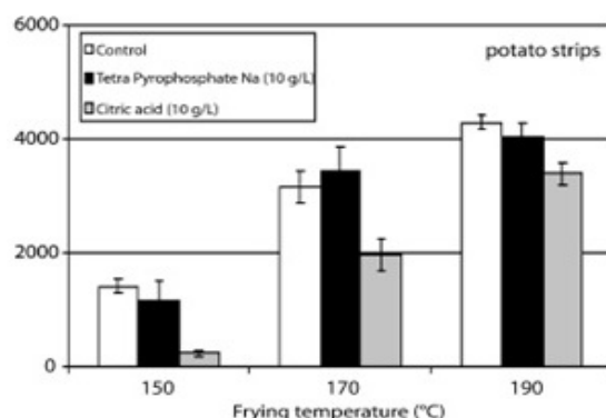
شکل ۵. اثر اسید سیتریک و تترا پیرو فسفات سدیم بر میزان تشکیل آکریلامید در چیپس سیب‌زمینی بر حسب \mu\text{g/kg} (محور عمودی)
