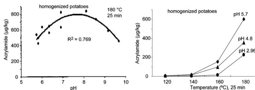
شکل ۸. اثر pH بر میزان تشکیل آکریلامید
