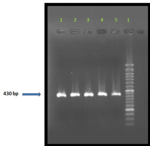
شکل 1. الگوی محصول PCR مربوط به PvuII ژن لیپوپروتئین لیپاز و مشاهده باند 430bp در تمامی نمونه‌های تکثیر یافته. L = مارکر 50bp می‌باشد.
